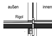
Schnitt durch Balkon-Terrassentür
